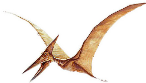
Pteranodon
